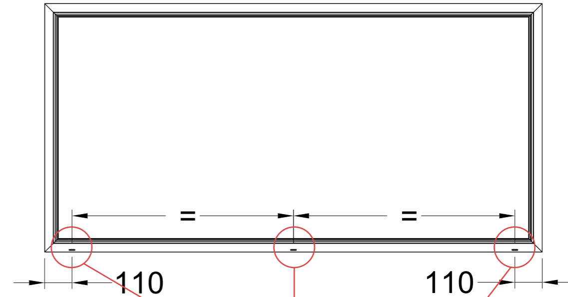
門框全圖
