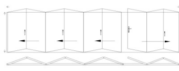
複合型 法式 摺疊門 963
