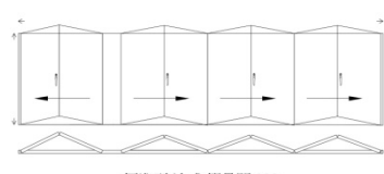
標準型 法式 摺疊門 826
