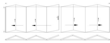
複合型 法式 摺疊門 954
