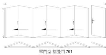
單門型 摺疊門 761
