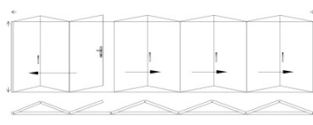
複合型 法式 摺疊門 936
