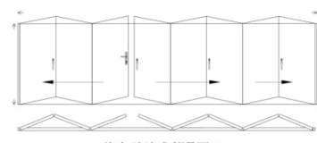
複合型 法式 摺疊門 835
