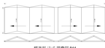
標準型 法式 摺疊門 844
