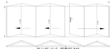
複合型 法式 摺疊門 743
