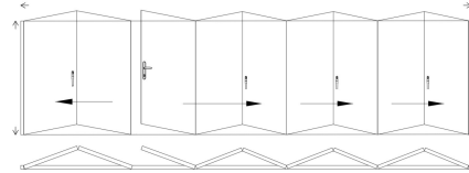
複合型 法式 摺疊門 927
