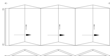
標準型摺疊門 606
