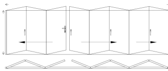
複合型 法式 摺疊門 835
