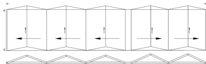
標準型 法式 摺疊門 1064
