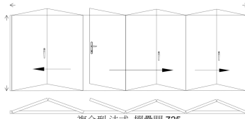
複合型 法式 摺疊門 725
