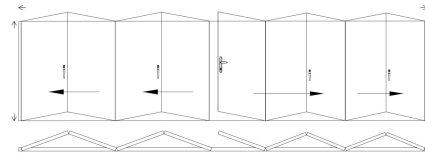
複合型 法式 摺疊門 945
