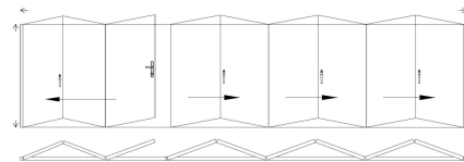
複合型 法式 摺疊門 936
