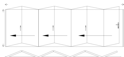
複合型摺疊門 770
