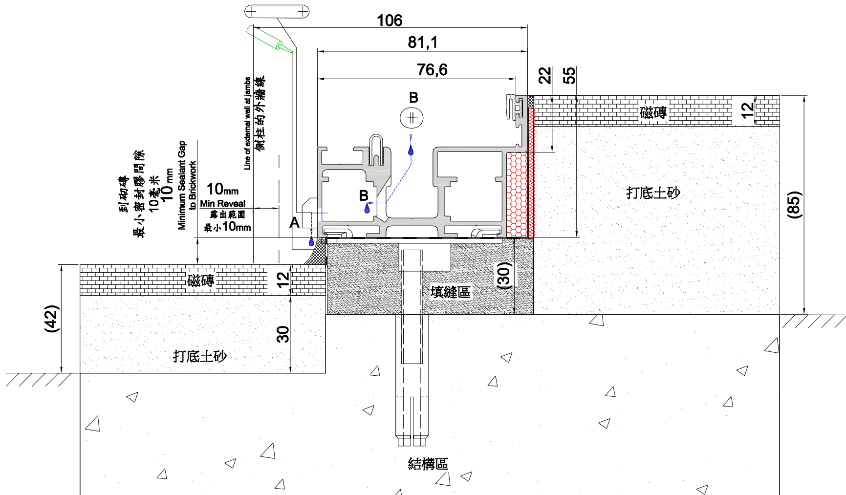
標準門檻施工示意圖 --- 濕式施工
